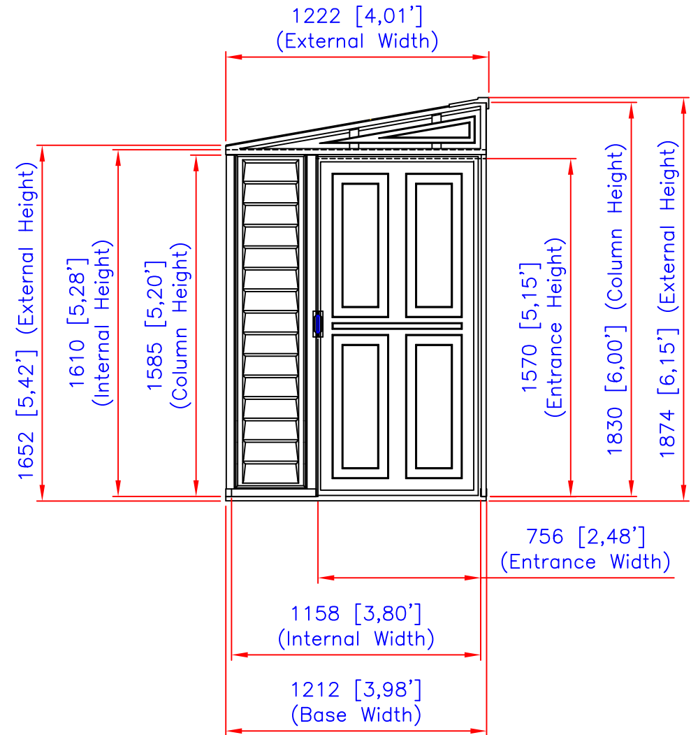
Elevation
