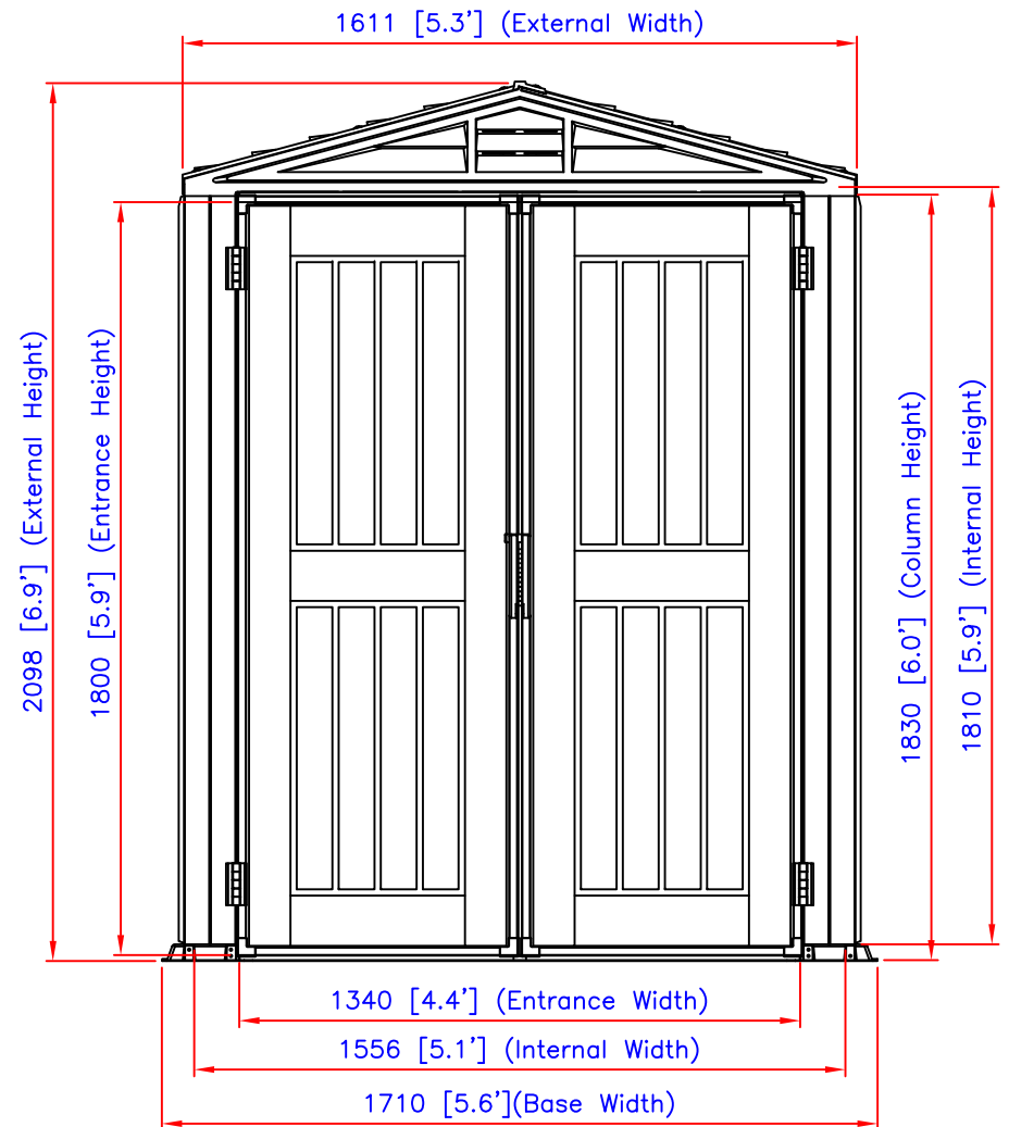
Elevation
